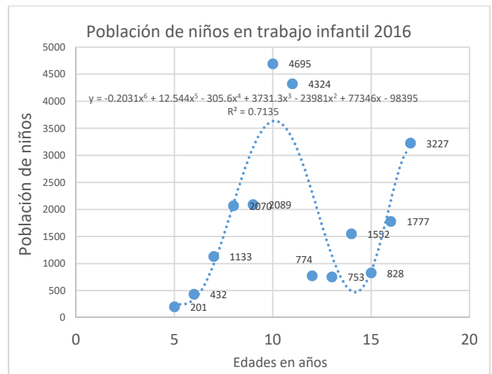
Figura 2. Diagrama de Dispersión para la encuesta de trabajo infantil durante el año 2016.
