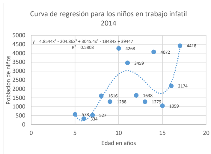
Figura 1. Diagrama de Dispersión para la encuesta de trabajo infantil durante el año 2014.
